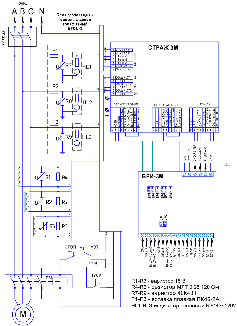
Рисунок 2 - Схема соединений станции управления погружным насосом СТРАЖ 3МС-95А
